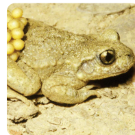
Alyte accoucheur
