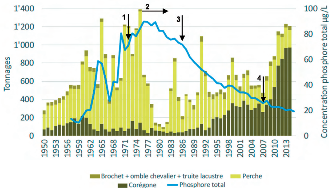
Figure 3.4. Évolution de la teneur en phosphore et de la composition des captures de poissons dans le lac Léman. 1 : démarrage de la déphosphatation dans les stations d'épuration ; 2 : diminution de la fertilisation phosphorée ; 3 : interdiction des phosphates dans les lessives en Suisse et baisse progressive des teneurs en France ; 4 : Interdiction des phosphates dans les lessives en France. D'après Mercier et al. , 2016.
