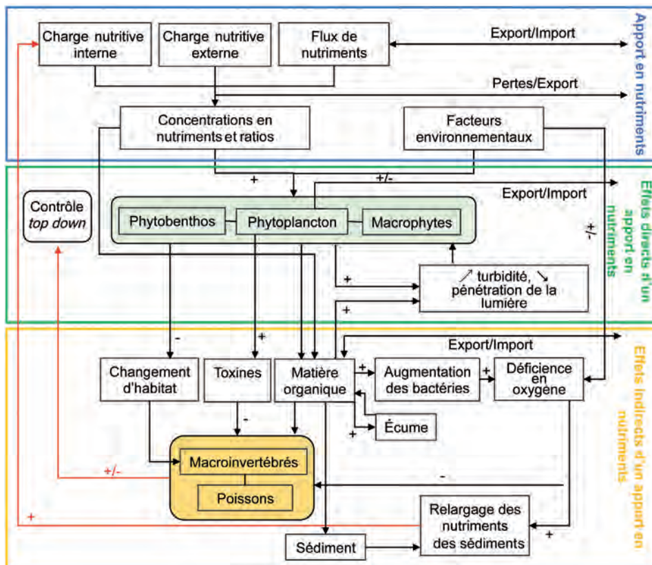
Figure 2.7. Schéma conceptuel de l'eutrophisation, pour tous les types de masses d'eau de surface. En rouge les rétrocontrôles. D'après Claussen et al. 2009.
