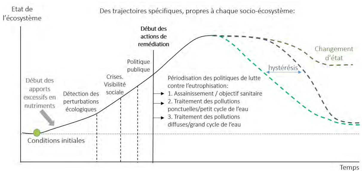
Figure 3.13. Périodisation de la lutte contre l'eutrophisation et réponses théoriques d'un écosystème. De nombreuses trajectoires sont possibles (linéaires ou abruptes, avec ou sans hystérésis, avec ou sans changement d'état), en fonction de l'histoire de l'écosystème aquatique, de ses caractéristiques physiques et biologiques ainsi que de celles de son bassin versant.
