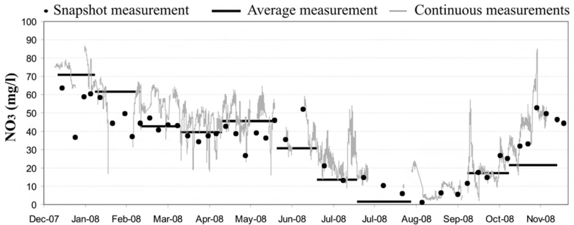
Figure 4.2. Comparaison de trois types de mesures des concentrations de \text{NO}_3^- , ponctuel, moyenné (SC Sampler) et continu. Source : Rozemeijer et al. , 2010. © American Chemical Society
