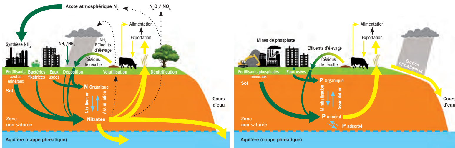
Figure 2.10. Cycles de l'azote (à gauche) et du phosphore (à droite).
