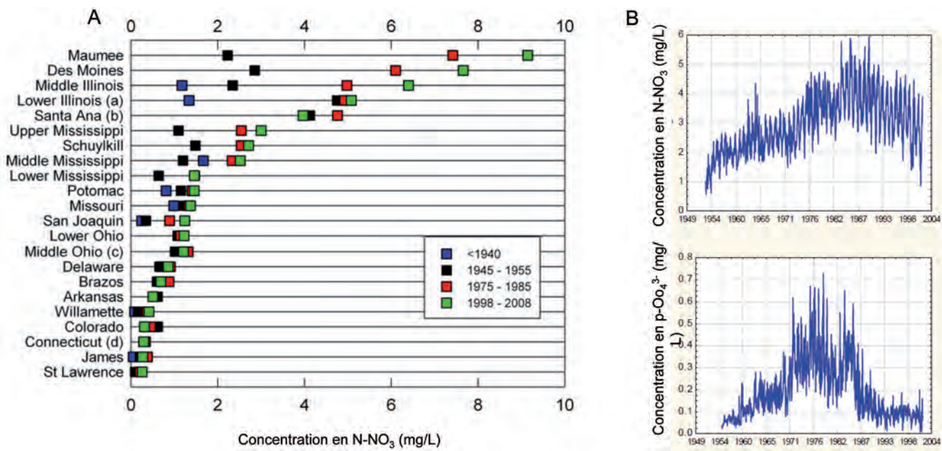
Figure 3.5. (A). Concentrations en nitrate de 22 rivières aux États-Unis (affluents du Mississippi, côte Est et côte Ouest), mettant en évidence l'enrichissement très précoce en nitrate. (B). Cinquante ans d'évolution du nitrate et du phosphate sur le Rhin. Sources : Stets et al. , 2015 ; Hartmann et al. , 2007.
