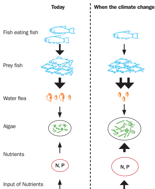
Figure 3.12. Évolution potentielle des structures trophiques sous hypothèse de changement global. Source : Jeppesen et al., 2014.
