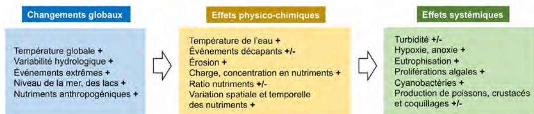
Figure 3.10. Principales composantes des effets cascades généralement décrits en réponse aux changements globaux projetés. D'après Paerl et al., 2014
