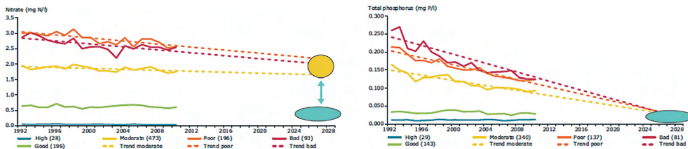
Figure 3.8. Tendances potentielles (2010-2027 en pointillé) pour l'azote et le phosphore, en valeur médiane dans chacune des catégories d'état écologique pour les eaux de surface européennes. Source : Werner, 2012. © European Environment Agency
