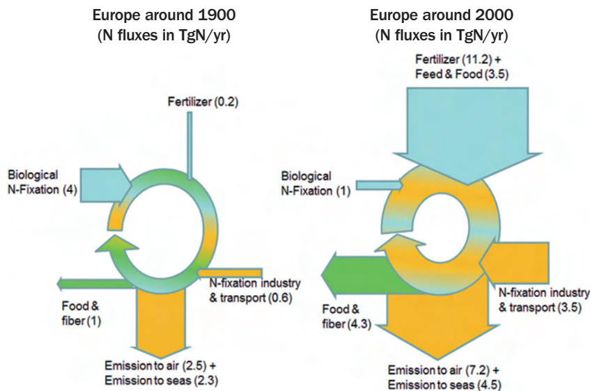
Figure 3.2. Évolution sur 100 ans du cycle de l'azote à l'échelle européenne. Source : Van Grinsven et al. , 2013. © American Chemical Society
