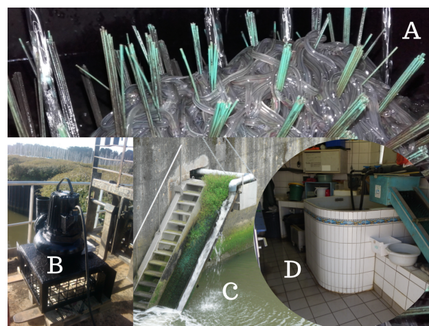
FIGURE 3: La passe à anguille du Gabion, passe principale 1996-2016.
