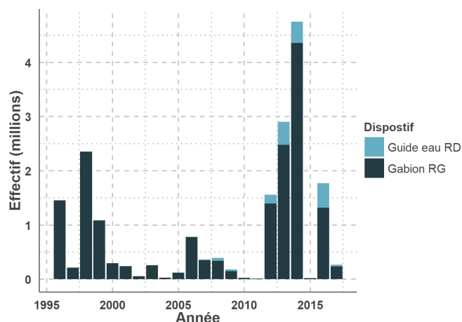
FIGURE 12: Effectif de civelles estimés sur les deux passes du barrage d'Arzal entre 1996 et 2017.
